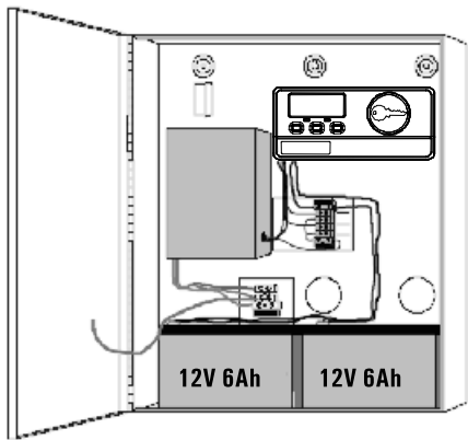
Boxed Easikey 250
